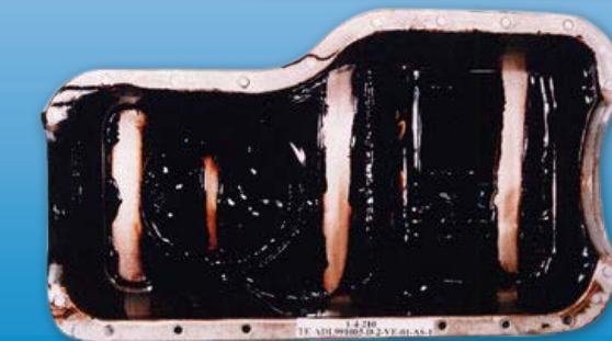
Motorenbauteil nach Standardtest mit Motorenöl ohne XMF® Technologie
